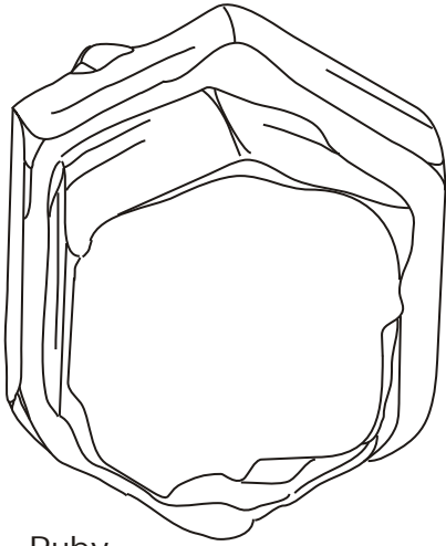
Ruby
